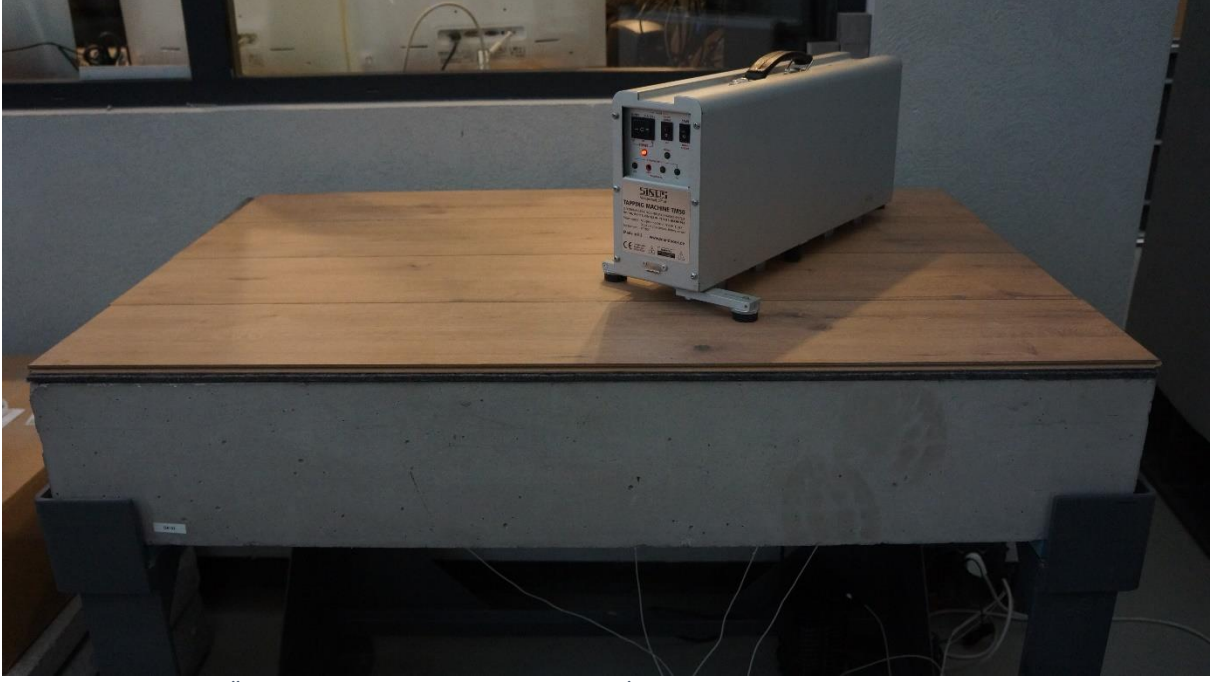
Şekil 4.2 Darbe Sesi Üreteci 1. Konumdayken Numune İle Beraber Deney Anı
