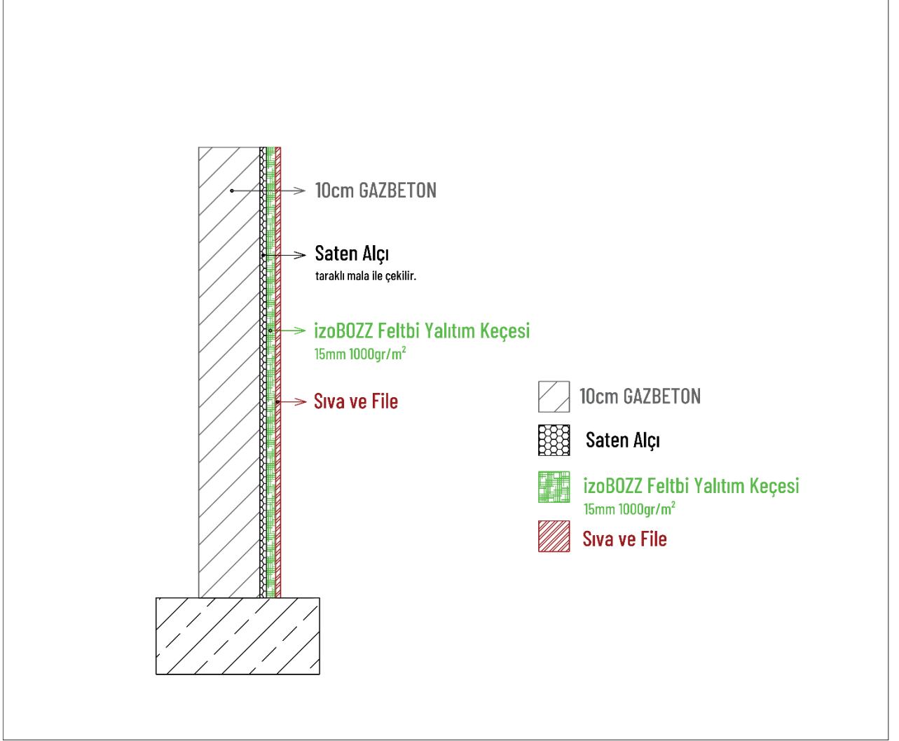
Şekil 3.1 Duvara ait teknik çizim
